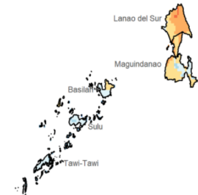
SPEI3 (Oct-Nov-Dec)
