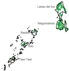
NDVI
